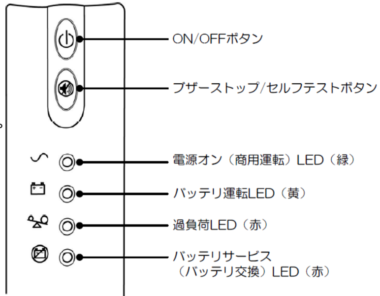
図 3-1 UPS フロントパネル
